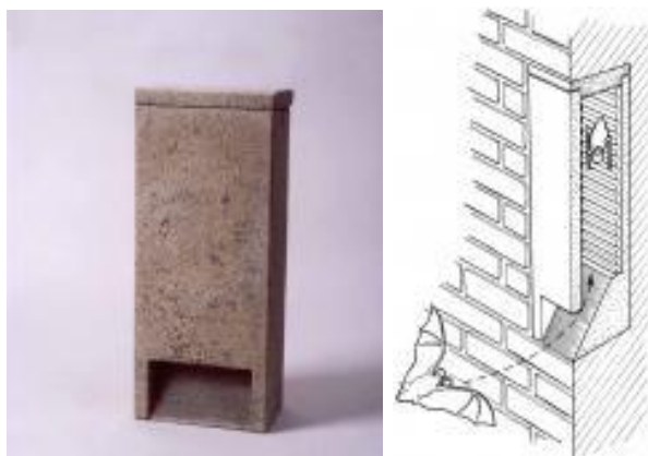
Obr. 9 Budka pro netopýry FR1 a její aplikace
